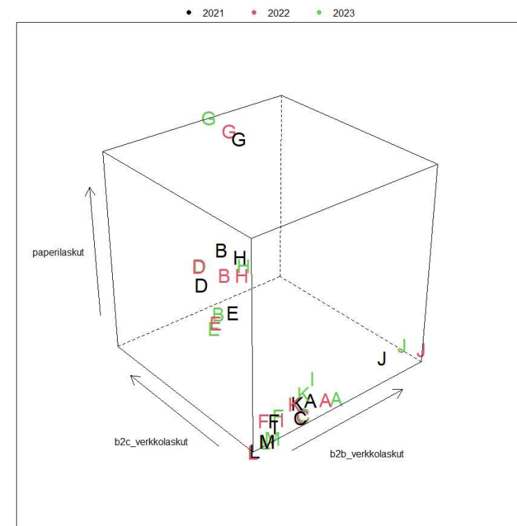
Operaattorikyselyn vastauskuutio
